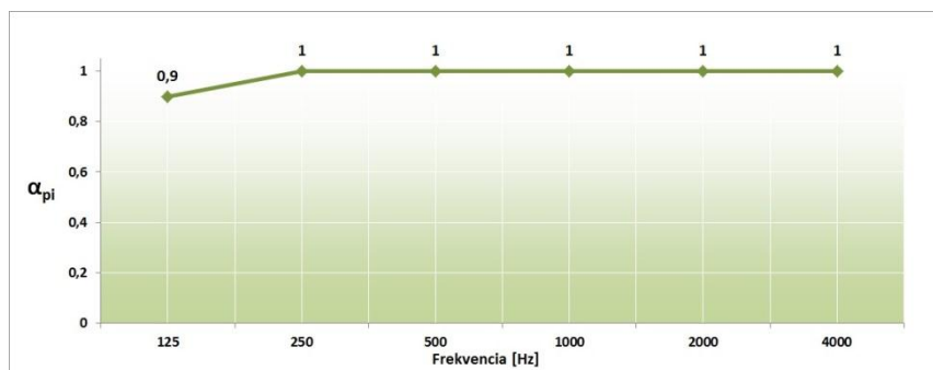
Priebeh činiteľa zvukovej pohltivosti pre OBIFON Diffsorber
