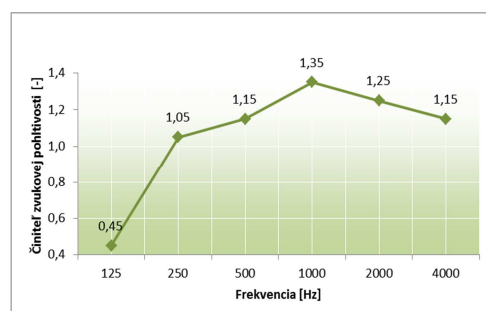
Priebeh činiteľa zvukovej pohltivosti pre OBIFON Basstrap stĺpovú pascu k
